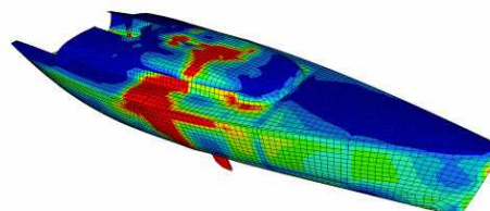
Foto 3: Analisi agli elementi finiti dell'AA38'
